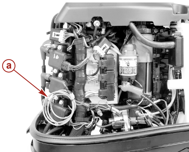
a - Напорная водяная труба
