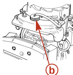
b - Крышка заливной горловины – Карбюраторные модели
