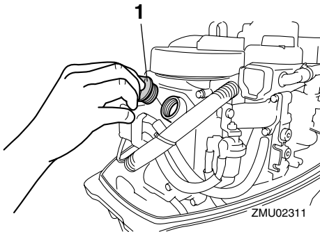
1. Крышка маслозаправочного отверстия
