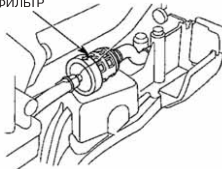
[1] ТОПЛИВНЫЙ ФИЛЬТР
