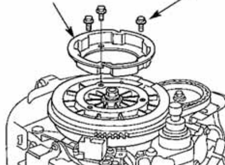
[1] ШКИВ СТАРТЕРА
