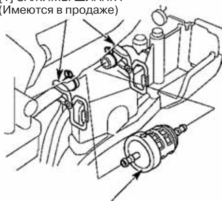
[2] ТОПЛИВНЫЙ ФИЛЬТР (В защитном кожухе)
