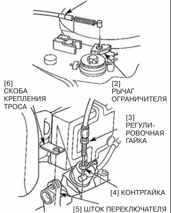
[1] ТРОС ВКЛЮЧЕНИЯ НЕЙТРАЛИ ПРИ ЗАПУСКЕ
