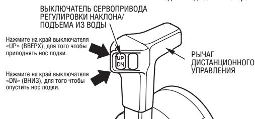
Пост управления спаренными подвесными моторами
